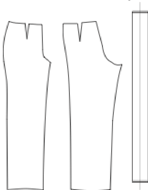
Детали кроя брюк
